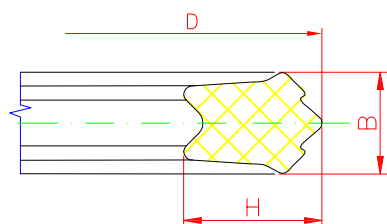
Tvar tesniaceho krúžku K- OD 200
